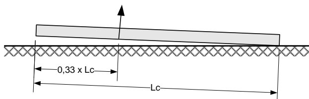
Rys. 2. Schemat pracy żelbetowego pala prefabrykowanego w czasie podnoszenia do kafara Prefabrykaty należy składować tak, aby nie powstawały w nich nadmierne naprężenia. Prefabrykaty powinny być podparte w sposób ciągły na wyrównanym podłożu lub punktowo na pryzmach z gruntu lub na podkładach drewnianych, co najmniej w miejscach uchwytów transportowych.
