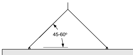
Rys. 1. Schemat pracy żelbetowego pala prefabrykowanego w czasie załadunku/rozładunku Przy podnoszeniu prefabrykatu do młota kafara należy wykorzystać jeden punkt zaczepienia w proporcjach 2:1 długości pala.
