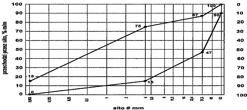
Rys. 7. Krzywe graniczne uziarnienia mieszanki kruszyw 0/63 mm do górnej warstwy podłoża ulepszonego
