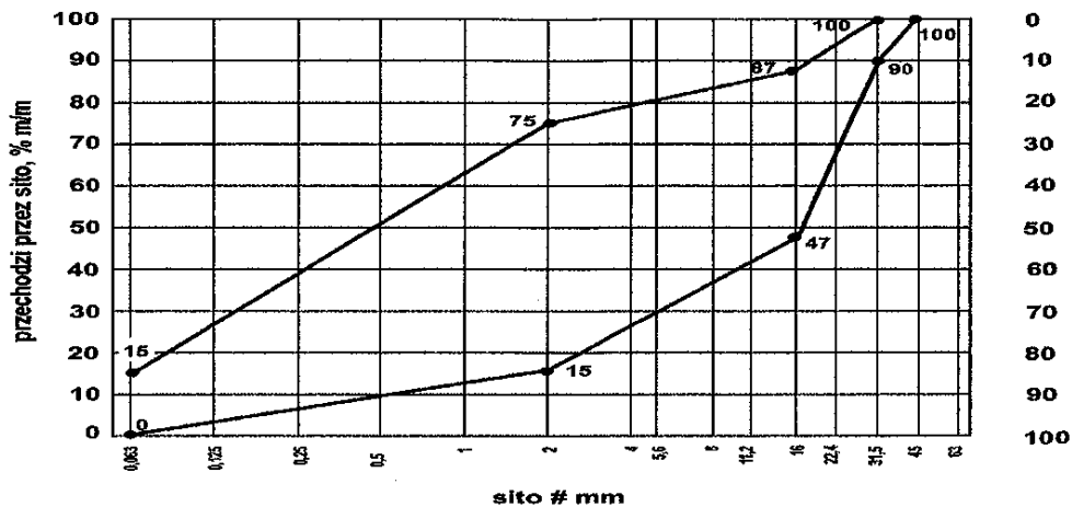
Rys. 5. Krzywe graniczne uziarnienia mieszanki kruszyw 0/31,5 mm do górnej warstwy podłoża ulepszonego
