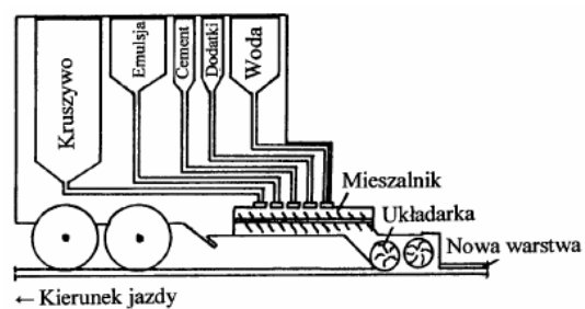
Rys. 1. Schemat urządzenia do rozkładania mieszanki mineralno-emulsyjnej
