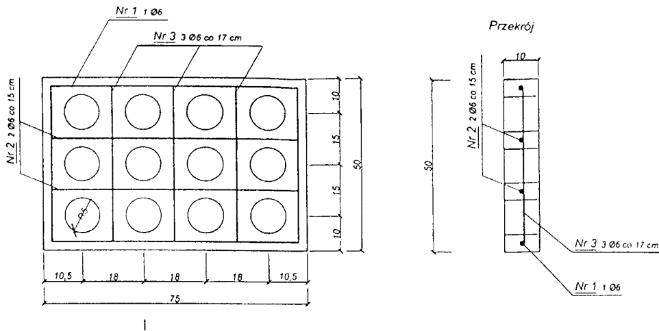
d) Płyta 0,75 × 0,50 × 0,10 m z otworami okrągłymi
