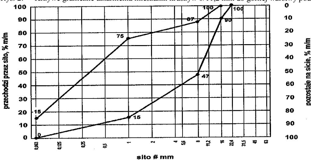
Krzywe graniczne uziarnienia mieszanki kruszyw 0/16 mm do górnej warstwy podłoża ulepszanego
