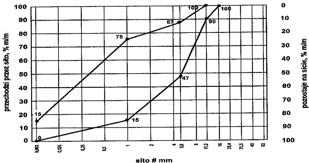
Krzywe graniczne uziarnienia mieszanki kruszyw 0/11,2 mm do górnej warstwy podłoża ulepszanego
