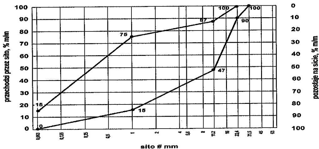
Krzywe graniczne uziarnienia mieszanki kruszyw 0/22,4 mm do górnej warstwy podłoża ulepszanego
