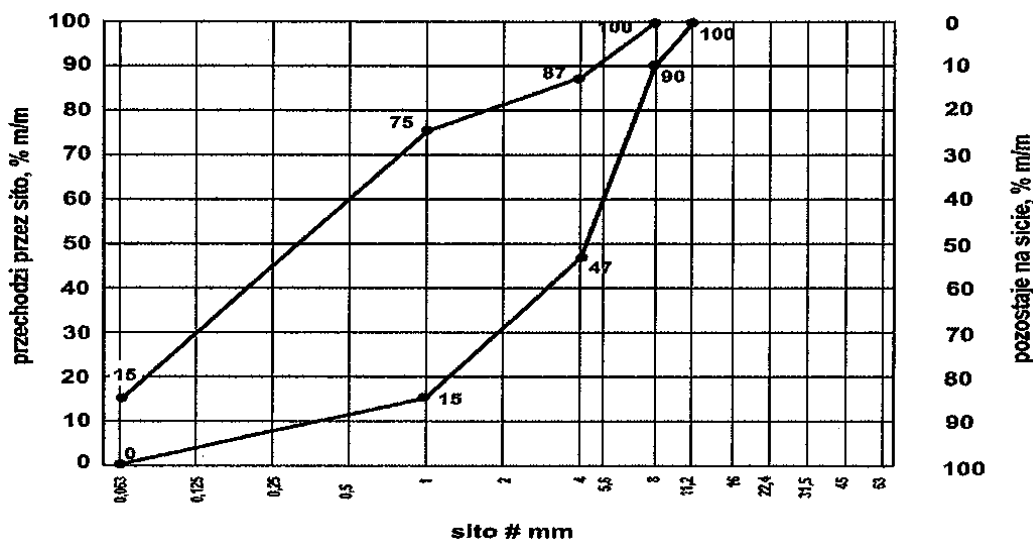
Rys. 1. Krzywe graniczne uziarnienia mieszanki kruszywo 0/8 mm do górnej warstwy podłoża ulepszonego
