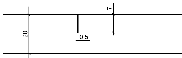
Szczelina nacięta w podbudowie (bez wypełnienia), na której będzie ułożona warstwa ściernala z mieszanki mineralno-asfaltowej
