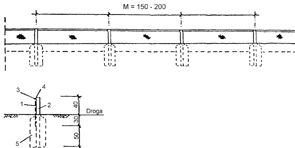
Rys. 2.2. Przykład konstrukcji z siatki ogrodzenia naprowadzającego płazy i gady do przepustu pod drogą
