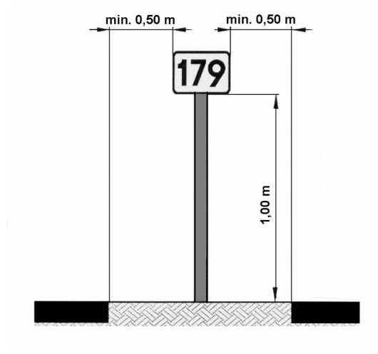
Rys. 4. Znak kilometrowy U-7 na samodzielny słupku
