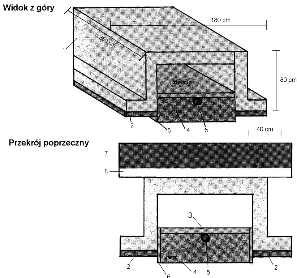
Rys. 2.1. Schemat konstrukcyjny przejścia dla płazów i gadów
