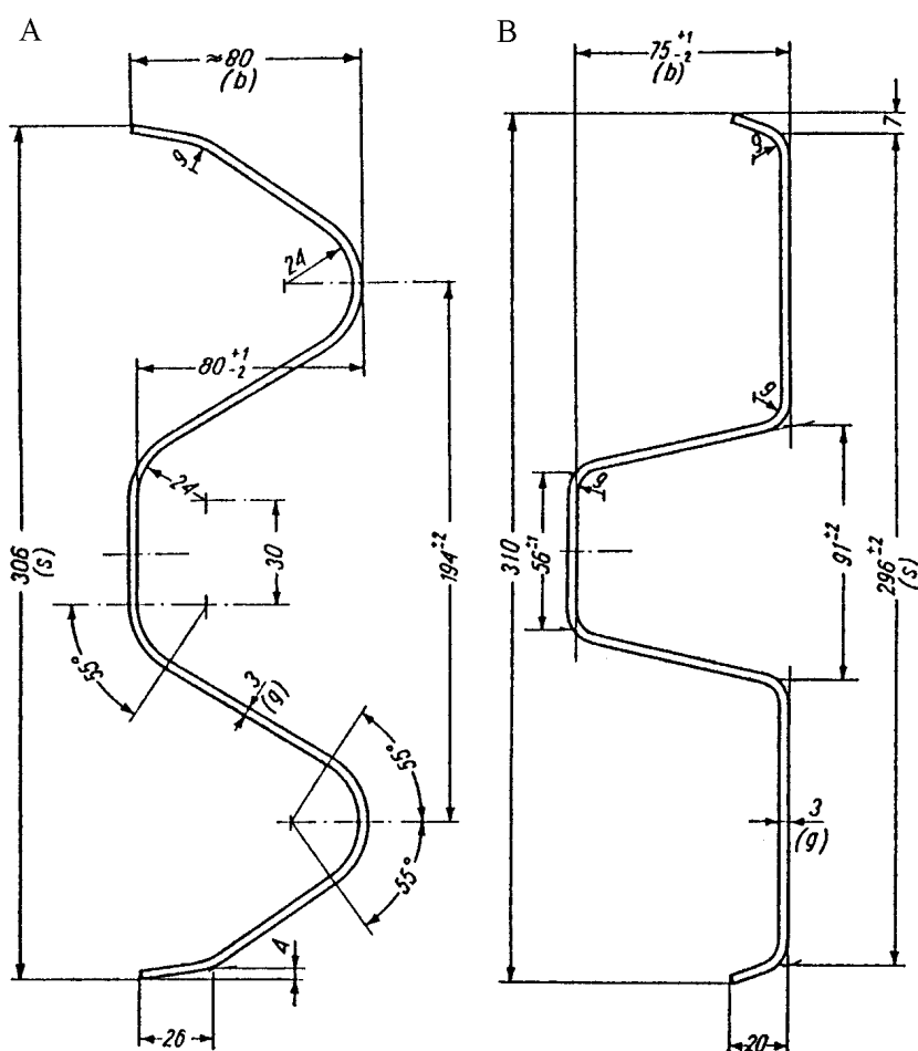
Załącznik 11.2 Bariery ochronne stalowe skrajne z prowadnicą z profilowanej taśmy
