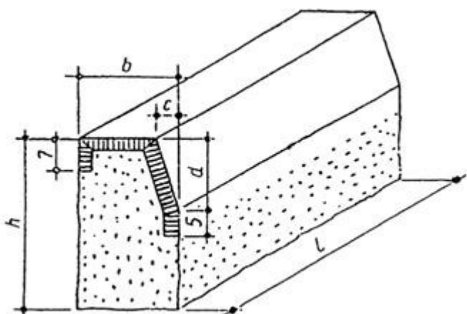
Wymiary krawężnika
