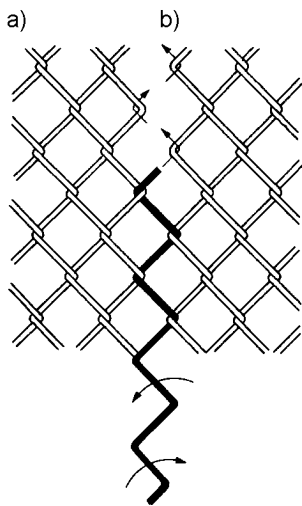
Rys. 3. Przykłady osadzenia słupków stalowych ogrodzenia w gruncie (wg [6]) a) Słupek osadzony w betonie ułożonym bezpośrednio w dołku b) Słupek osadzony w dołku po uprzednim oprawieniu go w bloczek betonowy
