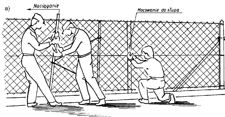
Rys. 9. Przykłady mocowania siatki do linek usztywniających (wg [6])
