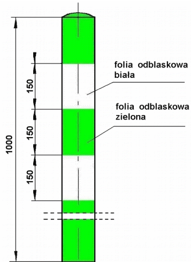
Rys. 2. Słupek prowadzący U-1b z naniesionym znakiem kilometrowym i hektometrym, przeznaczony do umieszczenia na barierze ochronnej, w hektometrze zerowym
