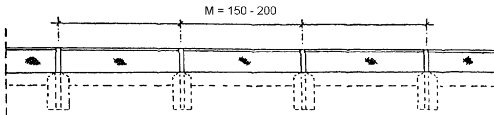
Rys. 2.2. Przykład konstrukcji z siatki ogrodzenia naprowadzającego płazy i gady do przepustu pod drogą
