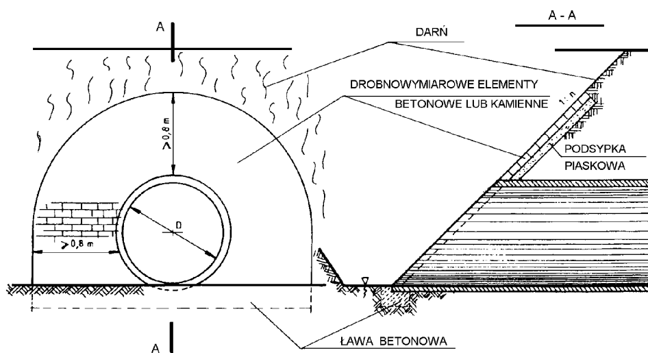
Rys. 10. Przykład umocnienia skarp przy wlocie przepustu za pomocą drobnowymiarowych elementów z betonowej kostki brukowej lub kamienia
