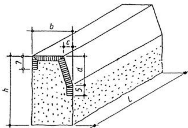
Wymiary krawężnika
