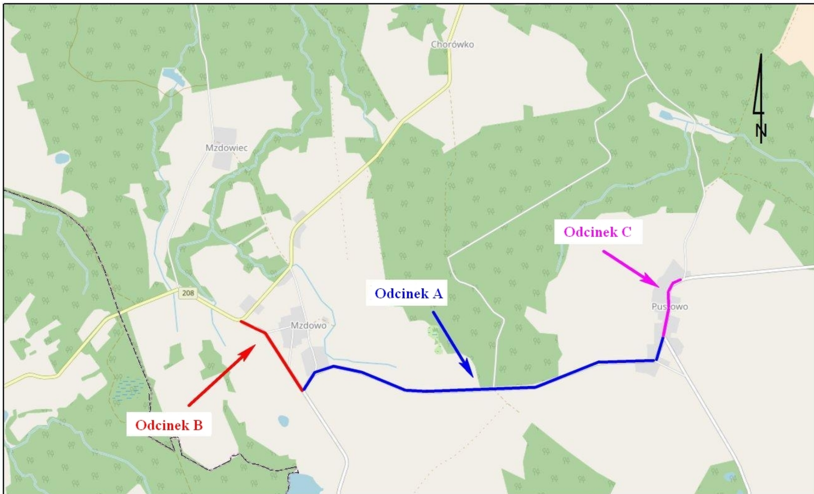
Plan orientacyjny lokalizacji inwestycji Przebudowa drogi powiatowej nr 1161G pomiędzy miejscowościami Mzdowo - Pustowo (Gmina Kępice)
